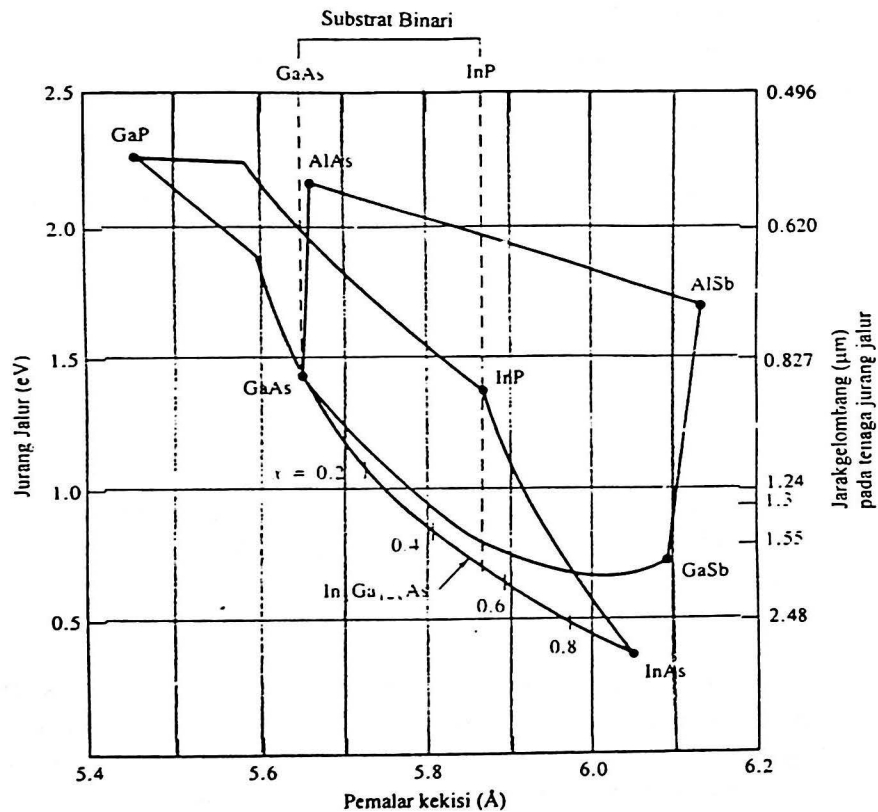
Rajah 1: Hubungan di antara Jurang Jalur dan Pemalar Kekisi bagi aloi dalam sistem \text{InGaAsP} dan \text{AlGaAsSb}
