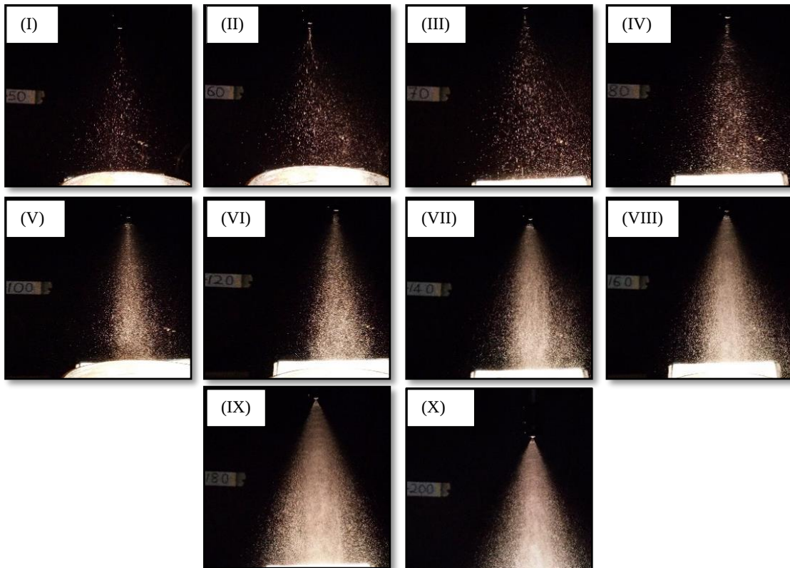
Figure 4.1(b): Injector 2 at (I) 50ml/min, (II) 60ml/min, (III) 70ml/min, (IV) 80ml/min, (V) 100ml/min, (VI) 120ml/min, (VII) 140ml/min, (VIII) 160ml/min, (IX) 180ml/min, (X) 200ml/min.
