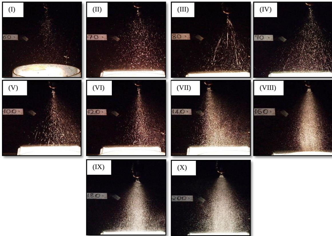
Figure 4.1(c): Injector 3 at (I) 60ml/min, (II) 70ml/min, (III) 80ml/min, (IV) 90ml/min, (V) 100ml/min, (VI) 120ml/min, (VII) 140ml/min, (VIII) 160ml/min, (IX) 180ml/min, (X) 200ml/min.
