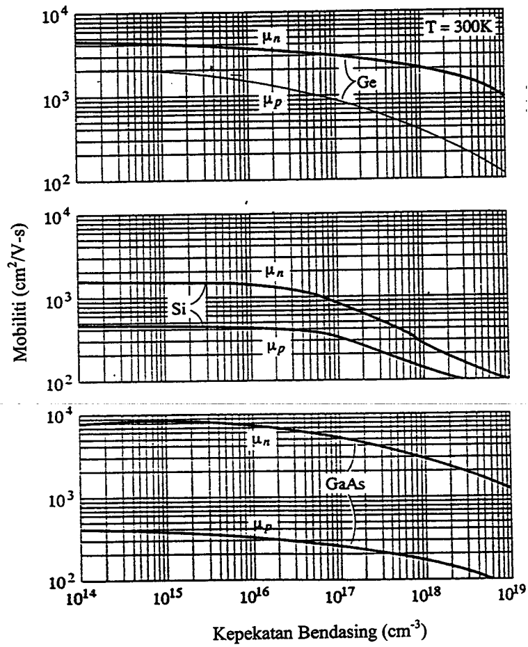
Pengaruh kepekatan bendasing terhadap mobiliti bagi elektron dan lohong pada suhu 300K bagi Ge,Si dan GaAs
