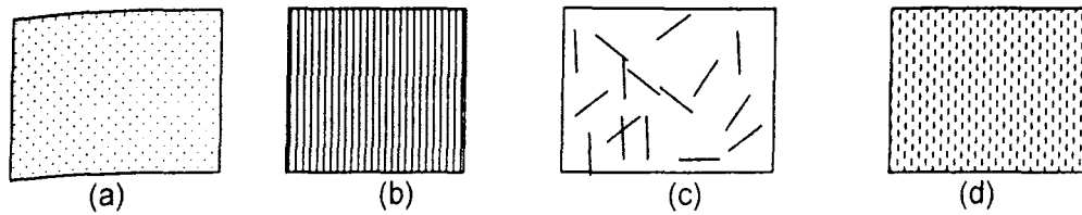
Rajah 2.3: Contoh-contoh komposit diperkuat partikel dan gentian (a) partikel secara rawak, (b) gentian selanjur secara eka arah, (c) gentian tidak selanjur secara rawak dan (d) gentian tidak selanjur secara eka-arah (Matthews & Rawlings, 1994).
