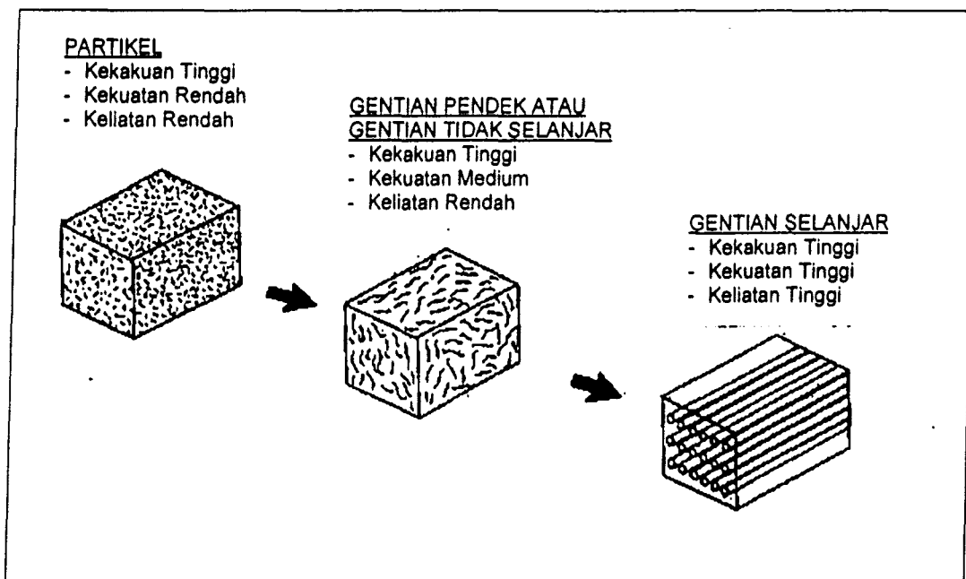
Rajah 2.9: Perbandingan sifat utama dalam KML (Textron, 1986).
