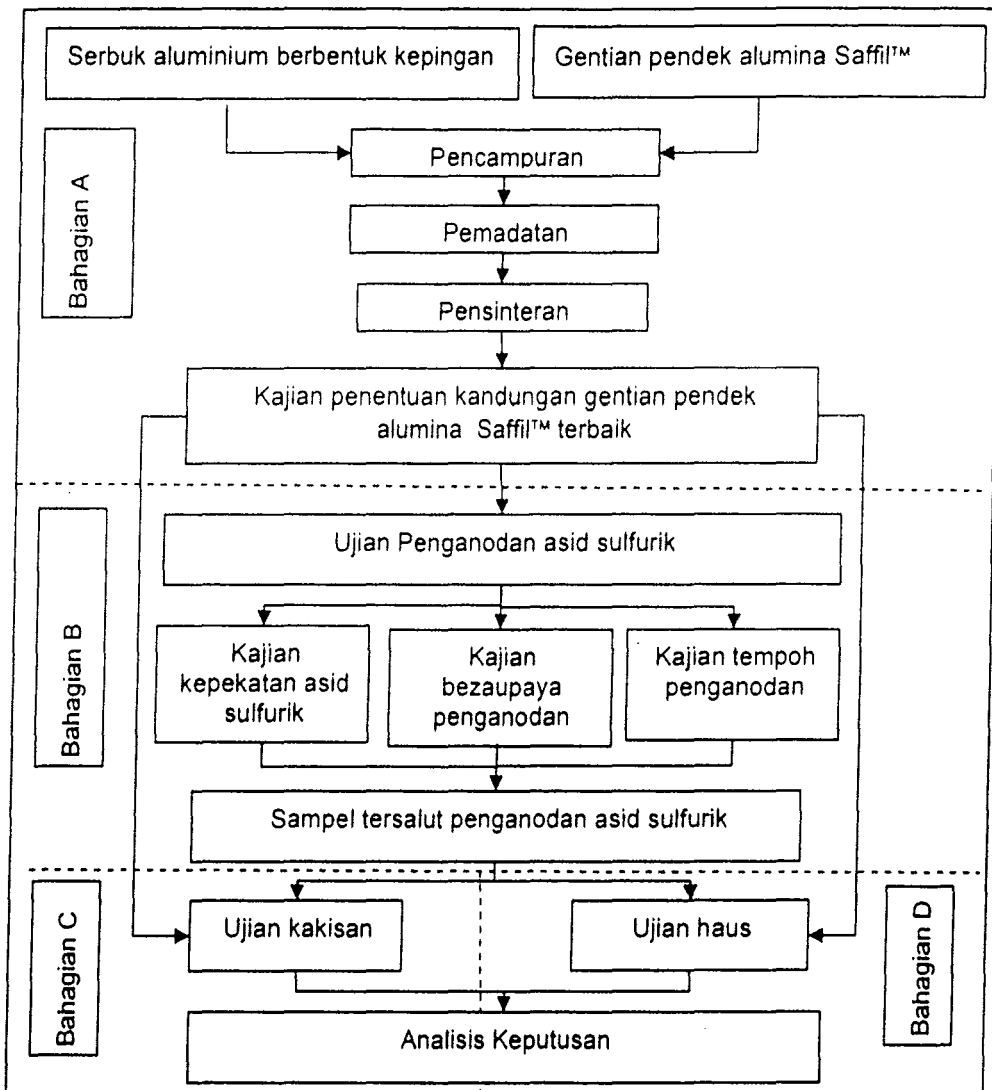
Rajah 1.2 Carta alir perjalanan penyelidikan yang terdiri daripada 4 bahagian eksperimen iaitu Bahagian A, Bahagian B, Bahagian C dan Bahagian D.
