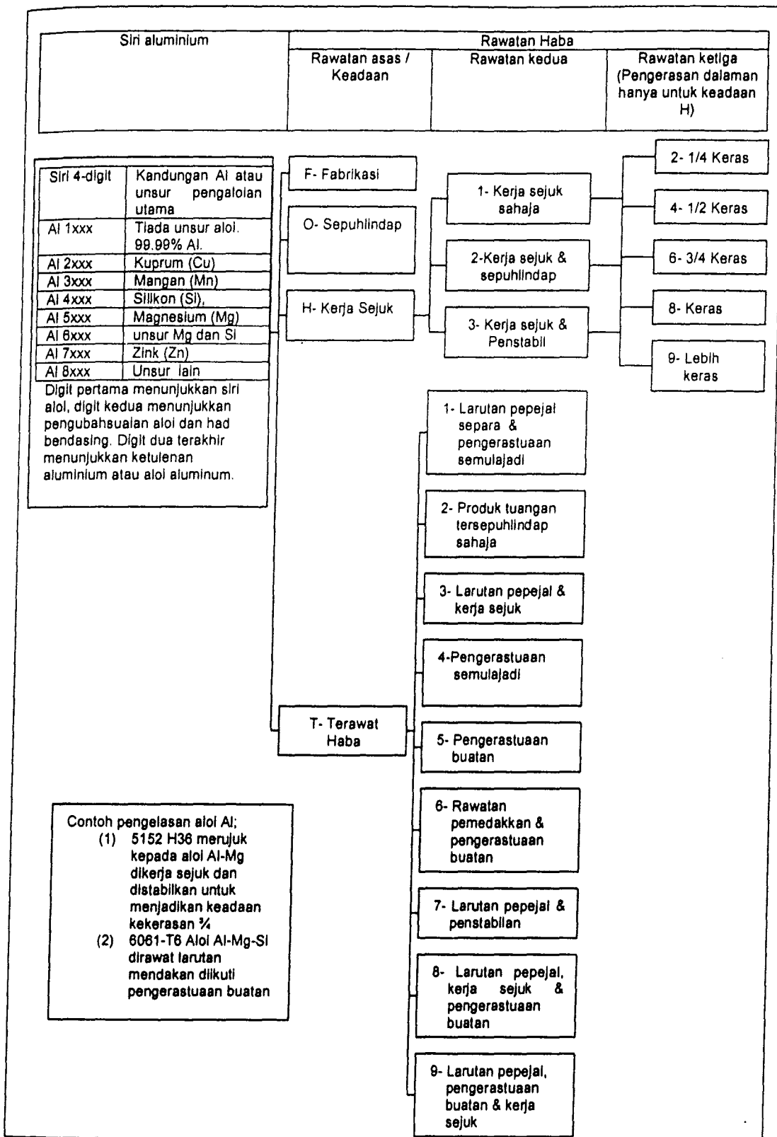
Rajah 1.1: Sistem pengelasan aloi Al dan rawatan haba (Polmear, 1995).
