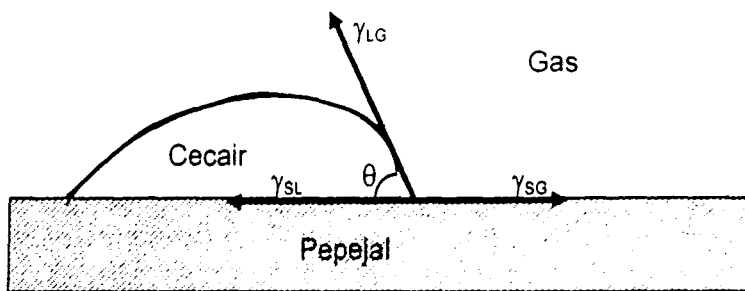
Rajah 2.4 Mekanisme penjerapan dan pembasahan (Matthews & Rawling, 1994).
