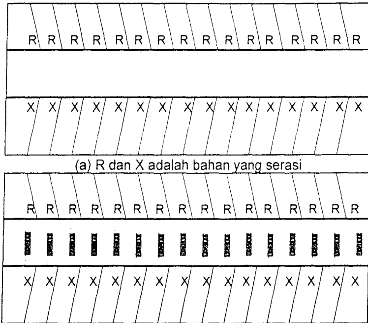
Rajah 2.7 Mekanisme pengikatan kimia (Matthews & Rawling, 1994).
