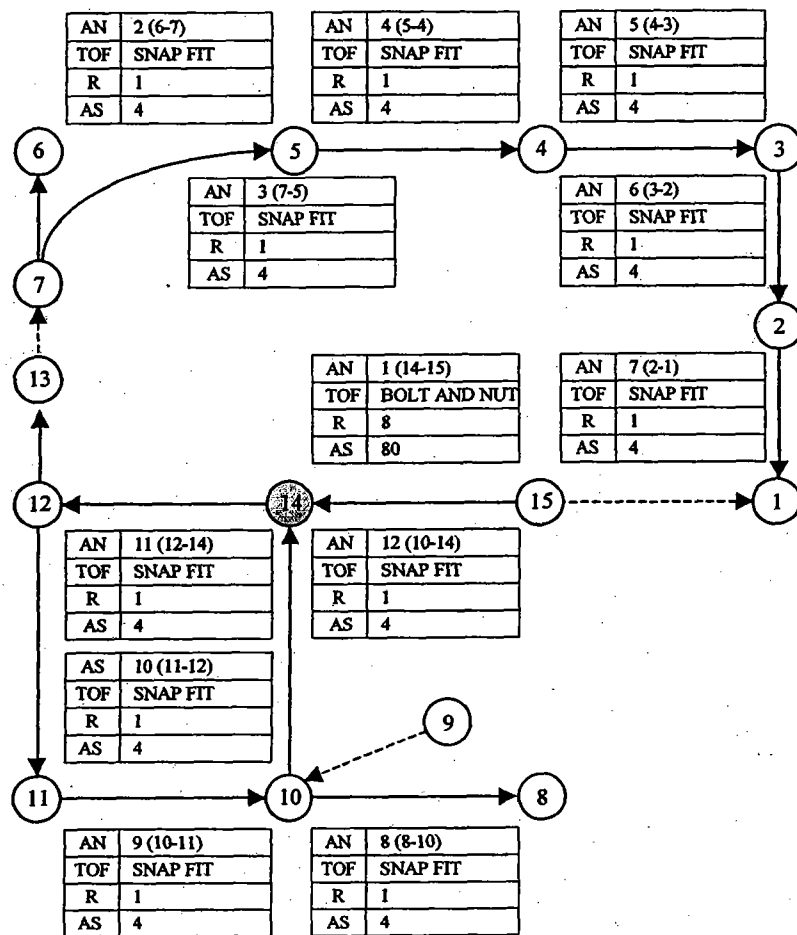
Rajah 6 Digraf peleraian komponen-komponen pam. Bulatan yang diwarnakan menunjukkan komponen yang terakhir dipasang dan yang pertama dileraikan
