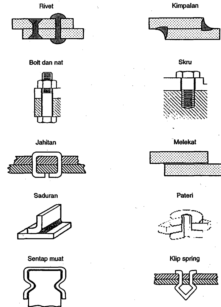
Rajah 1 Jenis-jenis pengikat [12, 13]
