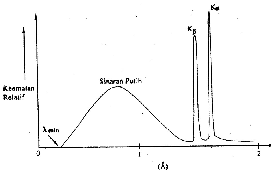
Rajah 1: Spektrum sinar-x bagi suatu sasaran tembaga (kuprum) secara skematik.
